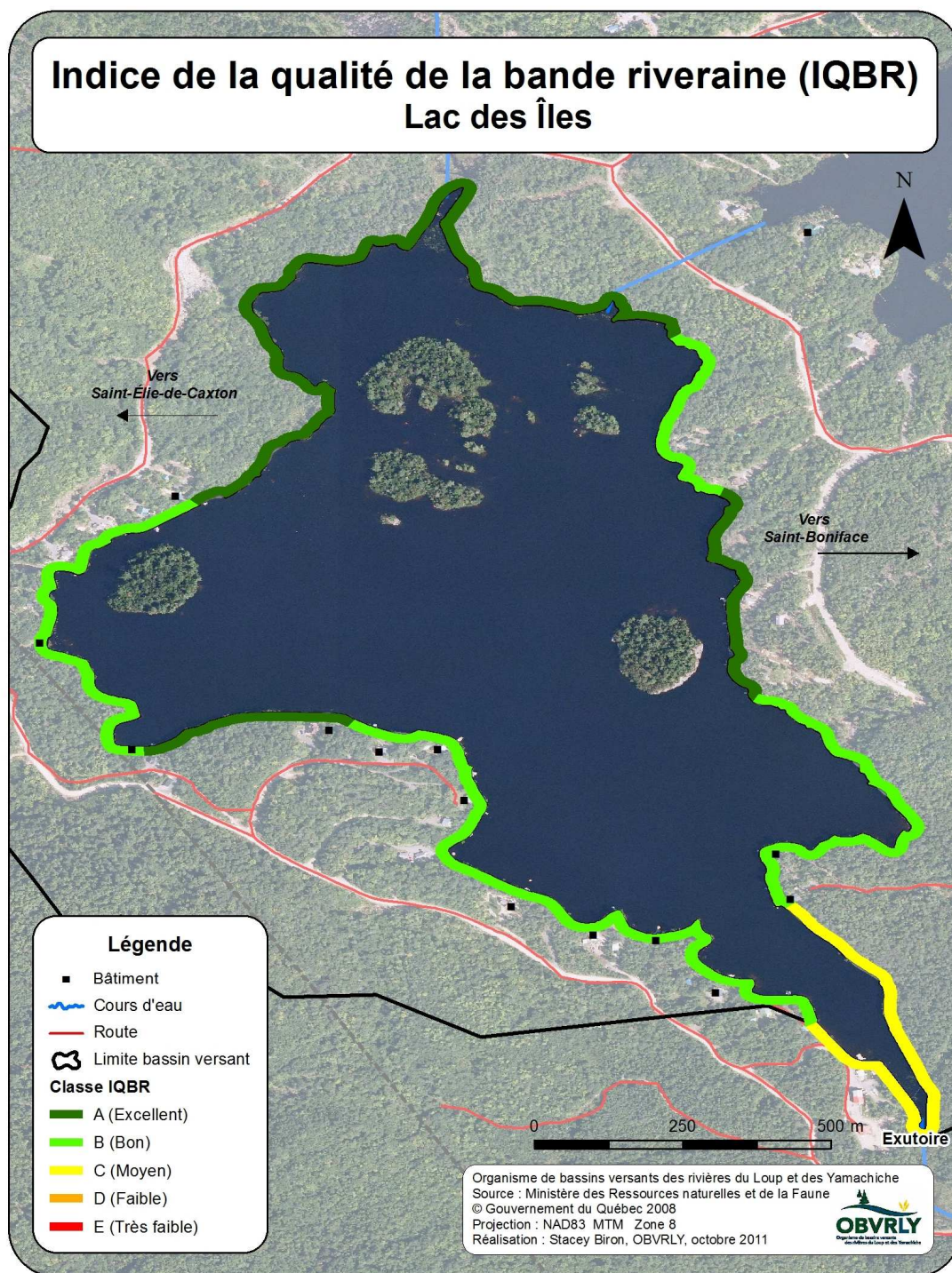
Carte 2 : Indice de la qualité de la bande riveraine (IQBR), lac des Îles, 2011
