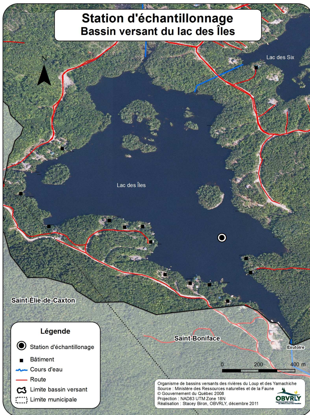
Carte 3 : Station d'échantillonnage des mesures effectuées à partir du protocole du Réseau de surveillance volontaire des lacs (RSVL) et des mesures des profils physico-chimiques, lac des îles - 2011
