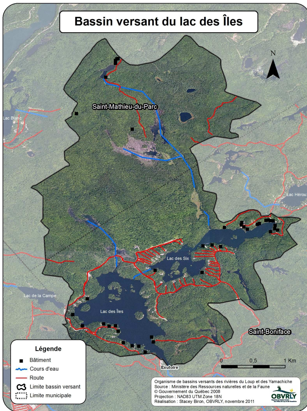
Carte 1 : Bassin versant du lac des îles, municipalité de Saint-Boniface
