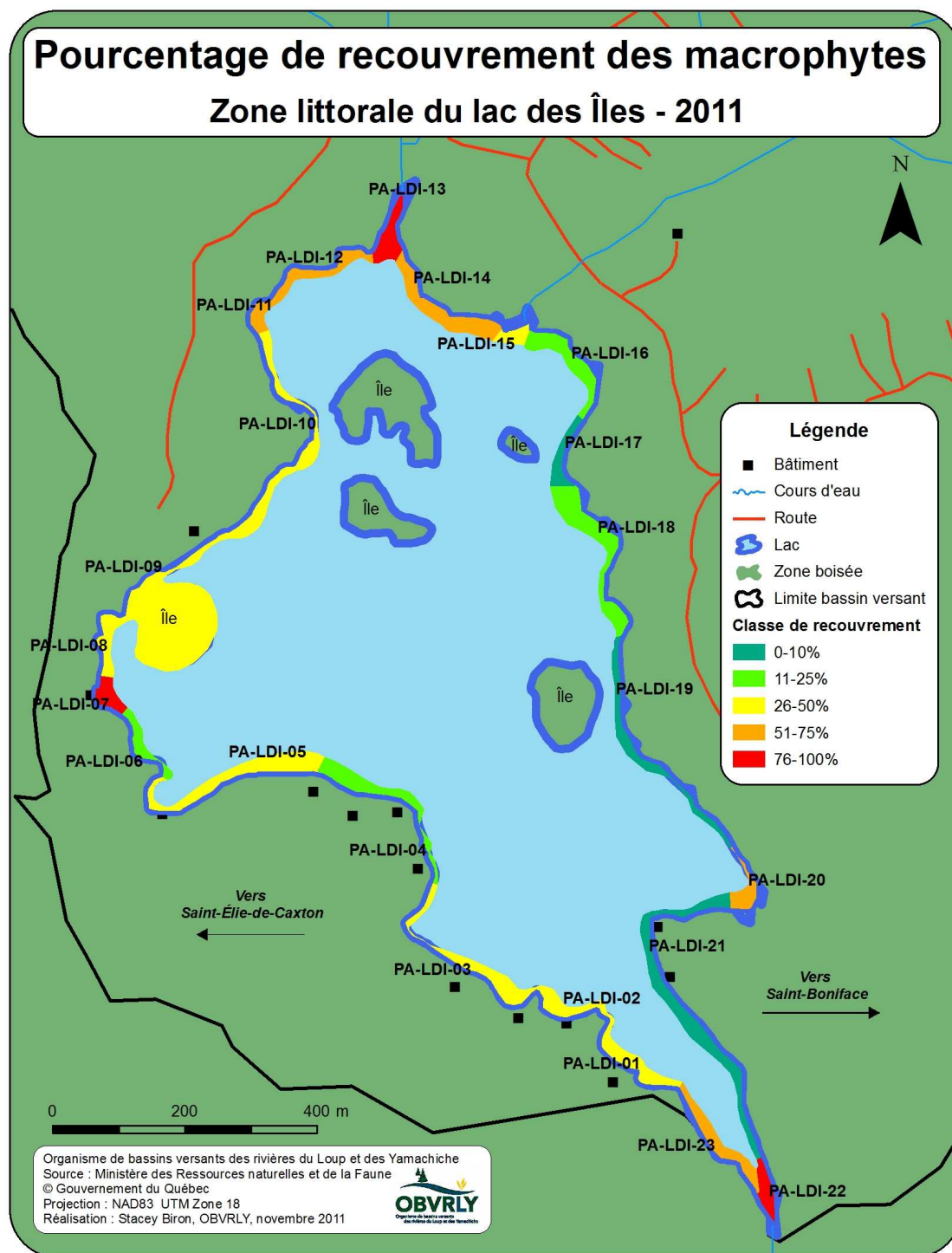
Carte 4 : Abondance des macrophytes, toutes espèces confondues, évaluée à partir du pourcentage de recouvrement des 23 secteurs inventoriés de la zone littorale, lac des îles - 2011
