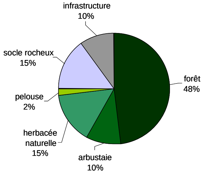
Figure 4 : Composition moyenne d'une rive appartenant à la classe C de l'IQBR, lac des Îles, 2011
