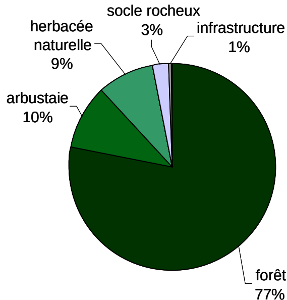
Figure 2 : Composition moyenne d'une rive appartenant à la classe A de l'IQBR, lac des Îles, 2011
