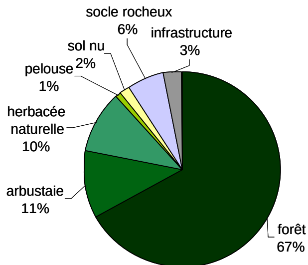
Figure 1 : Composition moyenne des rives du lac des Îles en 2011
