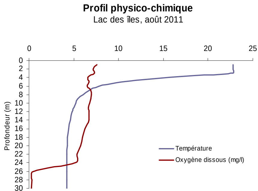
Figure 7 : Profil physico-chimique du lac des îles, août 2011
