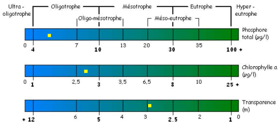
Figure 5 : Diagramme de classement du niveau trophique du lac des Îles obtenu à partir des moyennes estivales des données physico-chimiques en 2011 (tableau 3). Modèle de la figure tirée de : Réseau de surveillance volontaire des lacs (RSVL), MDDEP
