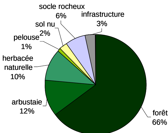
Figure 3 : Composition moyenne d'une rive appartenant à la classe B de l'IQBR, lac des Îles, 2011
